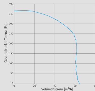
Druck-Volumen-Kennlinie UP-R
